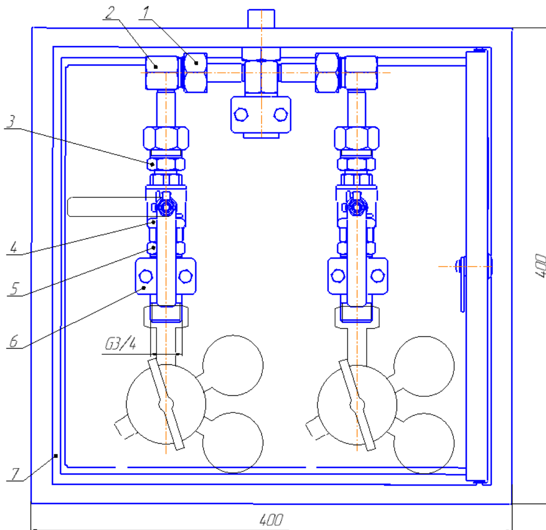
Рис.1 Пост газоразборный ПГК-50-3/2
